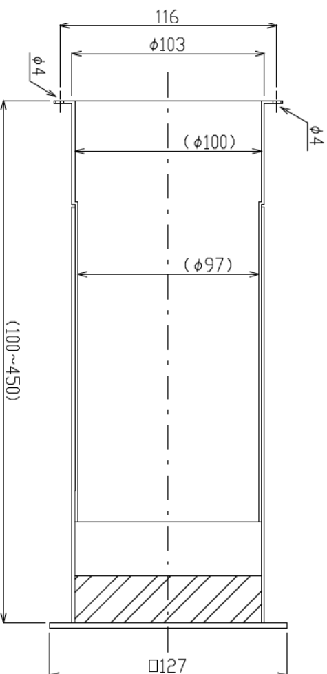
専用スリーブ (断面図)
